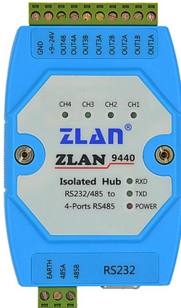
图 3 9440 接口图
