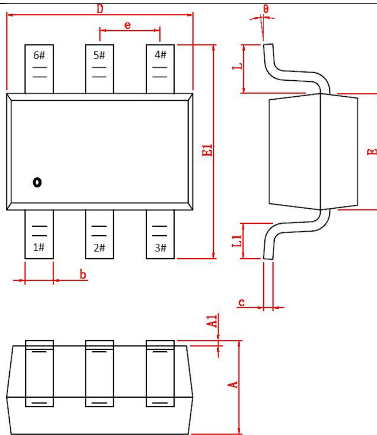
图 6 YOXO8110 尺寸图
