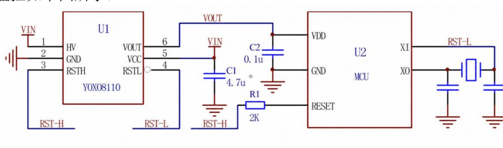
图 5 YOXO8110 电源监控示意图
