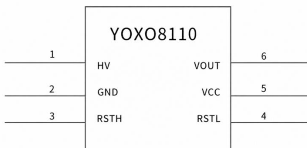
图 3 YOXO8110 封装
